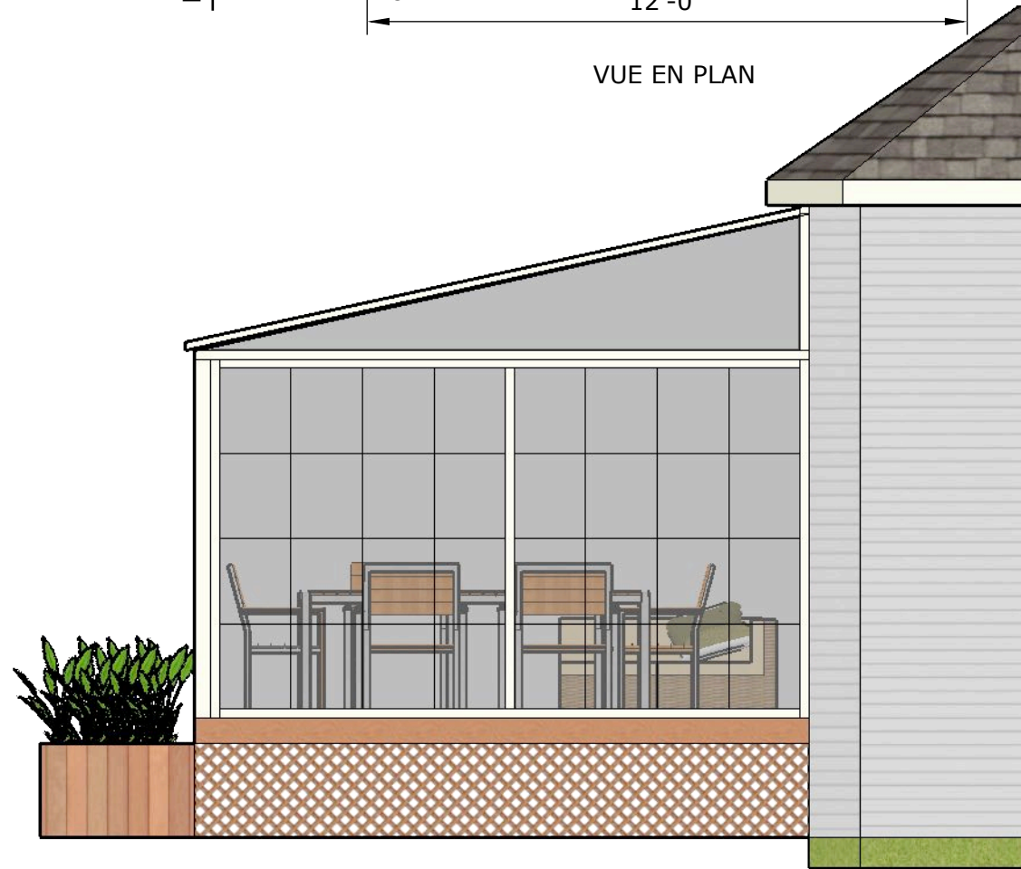
ÉLÉVATION DROITE
