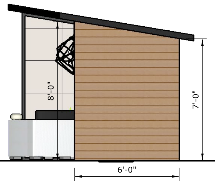
ÉLEVATION DROITE POOLHOUSE
